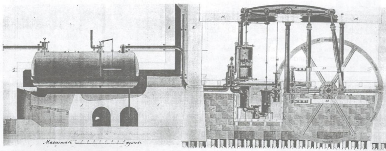
План паровой машины первой половины XIX века (ГАСО. Ф. 59. Оп. 3. Д. 1650. Л.3.)
